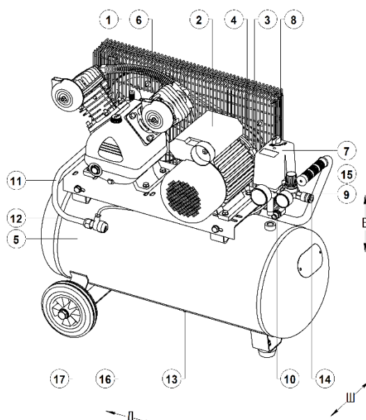
Рисунок 4 - Общий вид компрессора СБ4/С-50.LB24А
